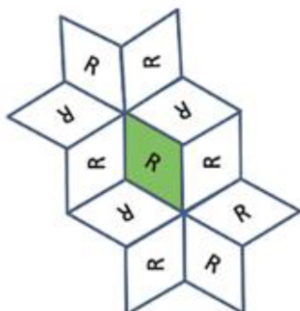
IUC 記号: p3 基本領域: 菱形
