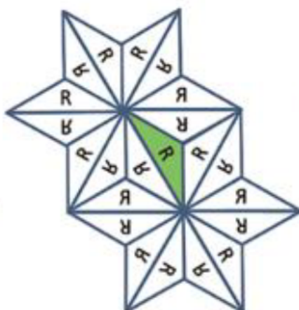
IUC 記号: p31m 基本領域: 二等辺三角形
