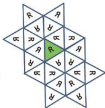
IUC 記号: p3m1 基本領域: 正三角形
