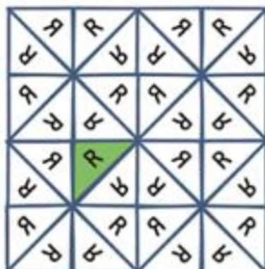
IUC 記号: p4m 基本領域: 二等直角三角形
