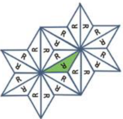
IUC 記号: p6 基本領域: 二等辺三角形
