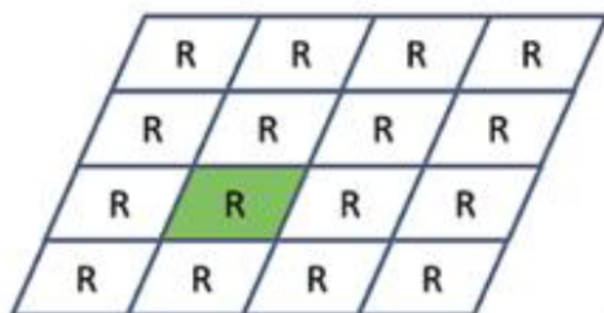
IUC 記号: p1 基本領域: 平行四辺形
