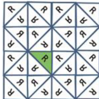
IUC 記号: p4g 基本領域: 二等直角三角形
