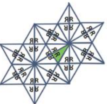
IUC 記号: p6m 基本領域: 正三角形の半分
