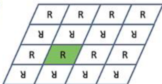
IUC 記号: p2 基本領域: 平行四辺形
