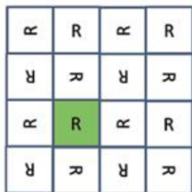
IUC 記号: p4 基本領域: 正方形
